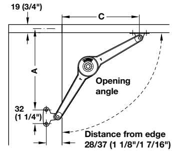
Lid Stay
